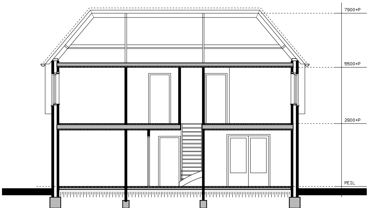
doorsnede 2
