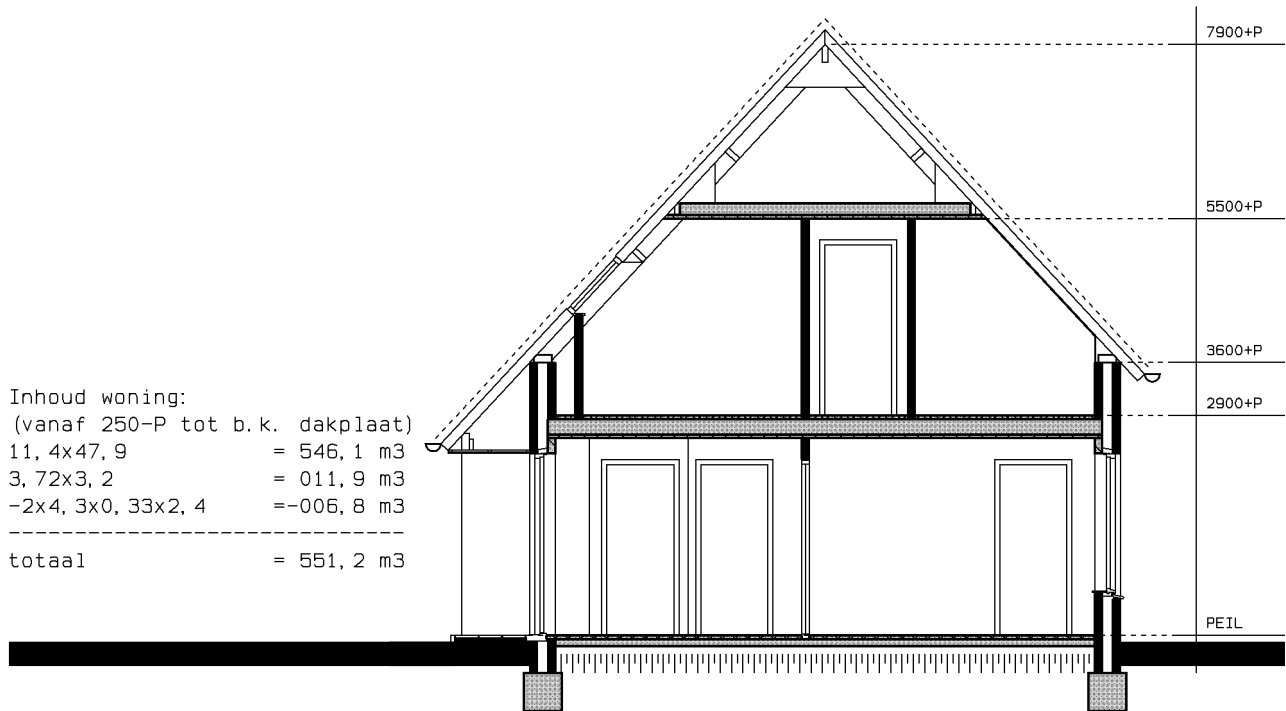
doorsnede 1
