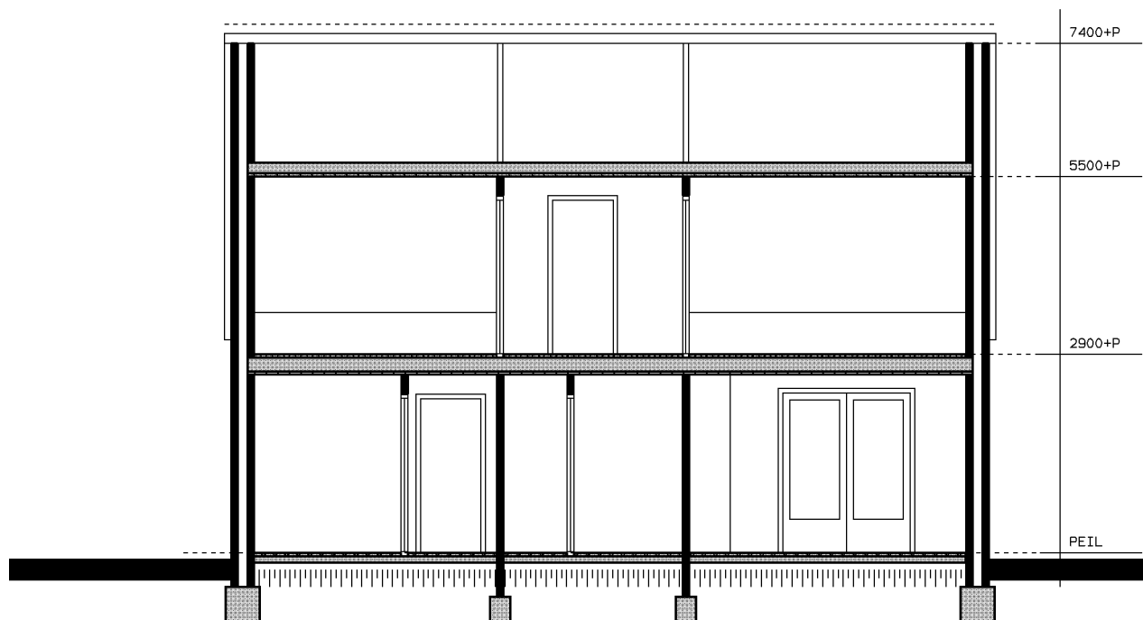
doorsnede 2
