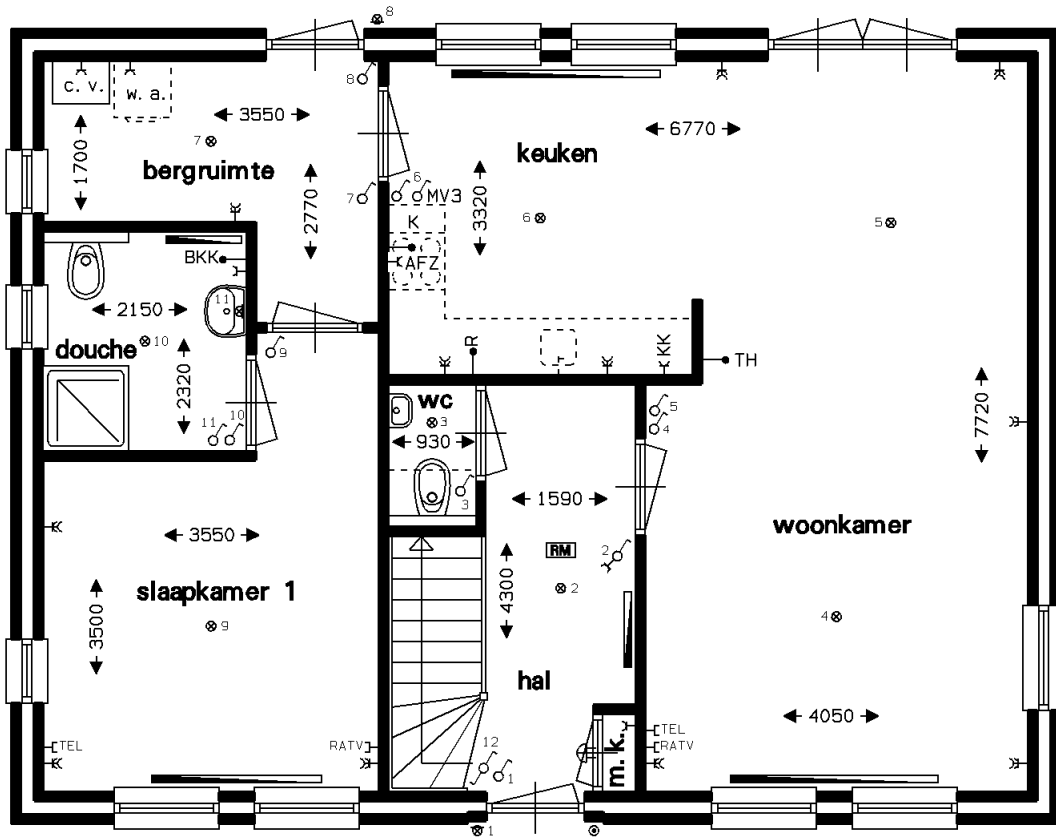
begane grond
