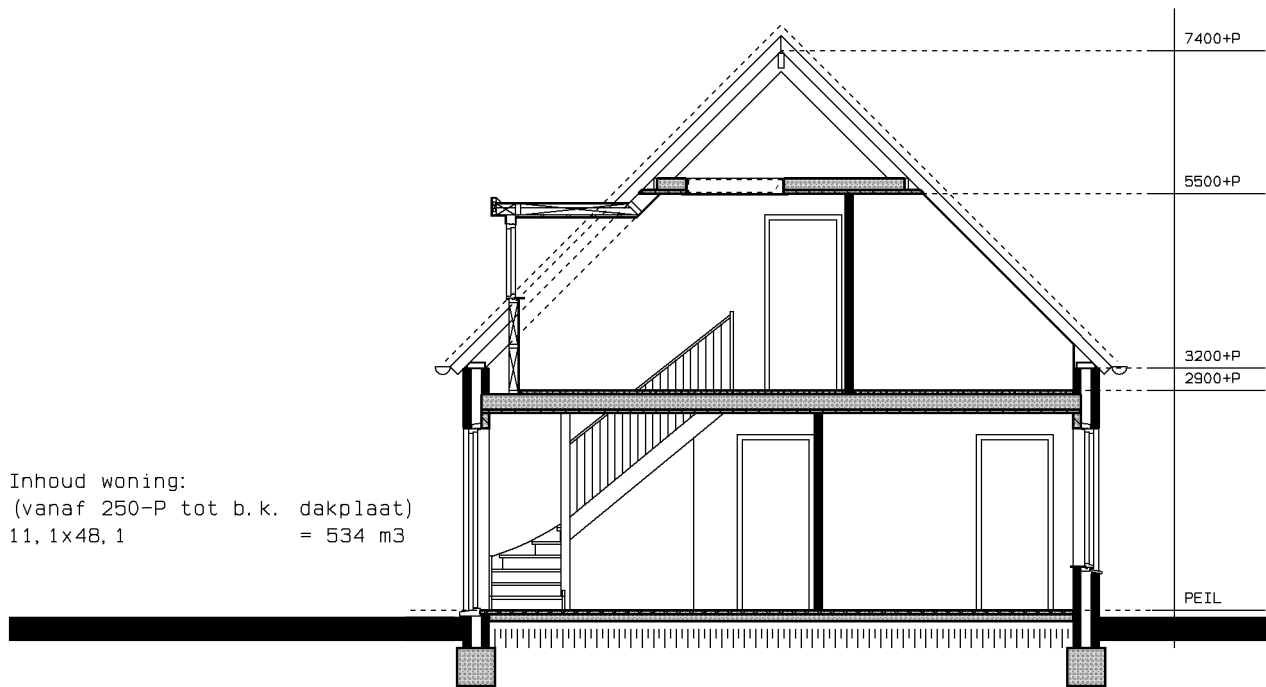
doorsnede 1
