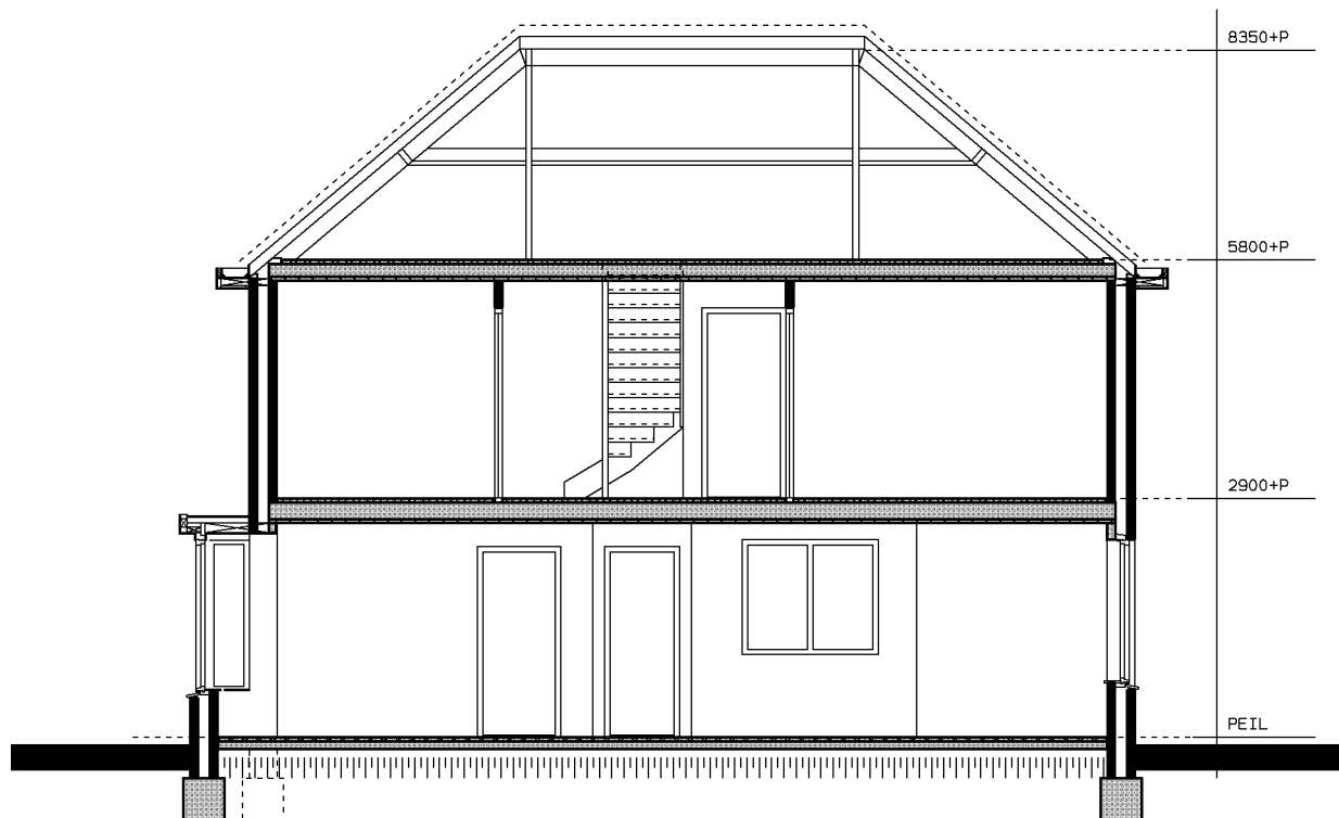
doorsnede 2
