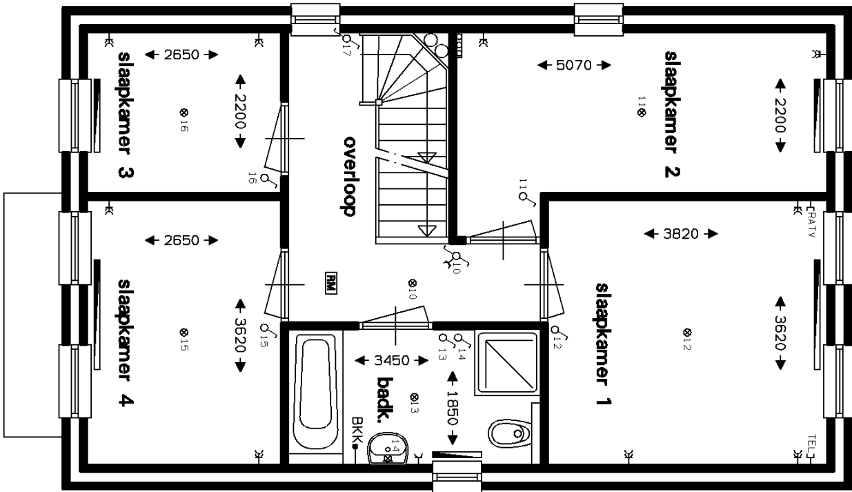
verdieping
