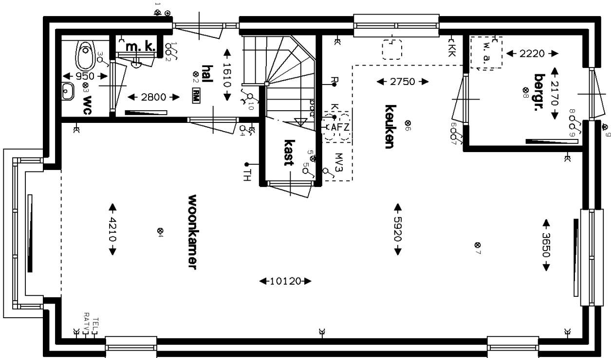
begane grond
