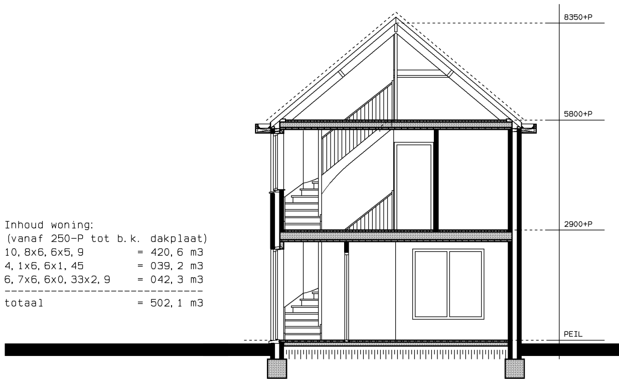
doorsnede 1
